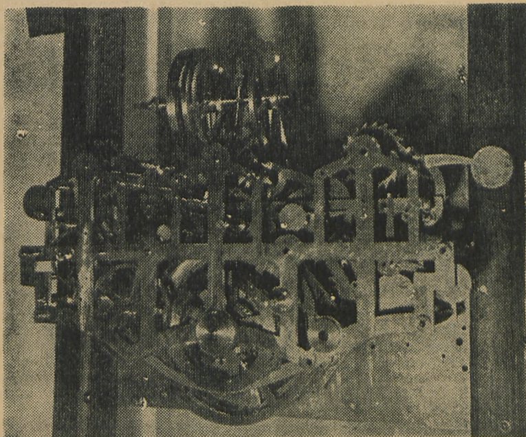
Dette værk arbejder kun 6 minutter om året — seks minutter i 12 nytårsnat falder det i slag og sørger for, at dagene i det kommende år falder på de rigtige datoer, og at månefaserne fastlægges rigtigt. Værket skal klare talt 570.000 kombinationer.
